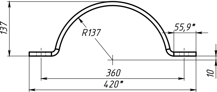
Поз.4 (Полухомут)
